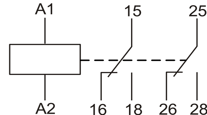
Рис. 3 5А ~ 250В, 5А = 30В
